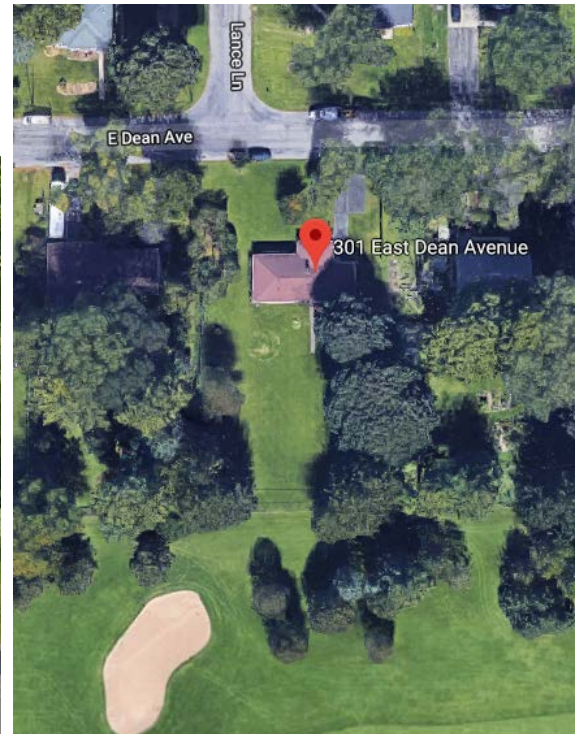
Google Earth
