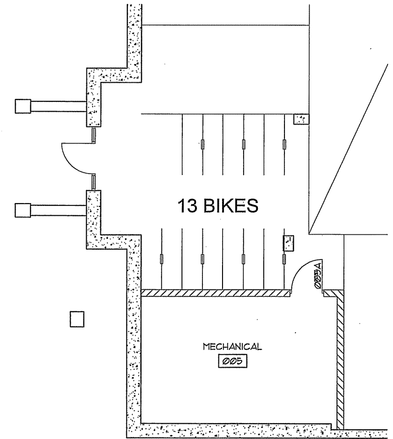
3 PLAN SCALE: 1/8" = 1'-0"
