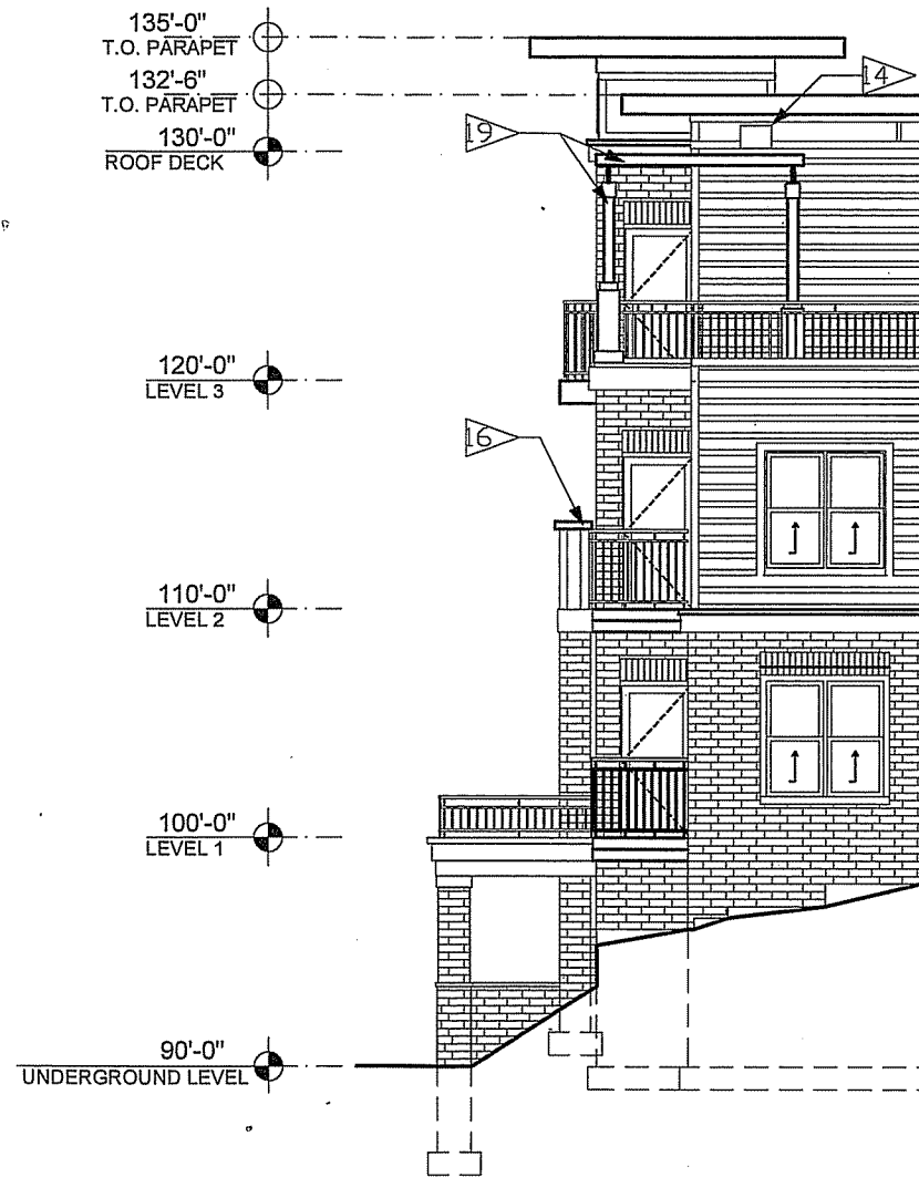
2 SOUTH ELEVATION SCALE: 1/8" = 1'-0"
