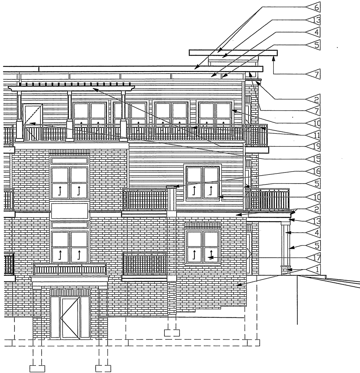
1 WEST ELEVATION SCALE: 1/8" = 1'-0"
