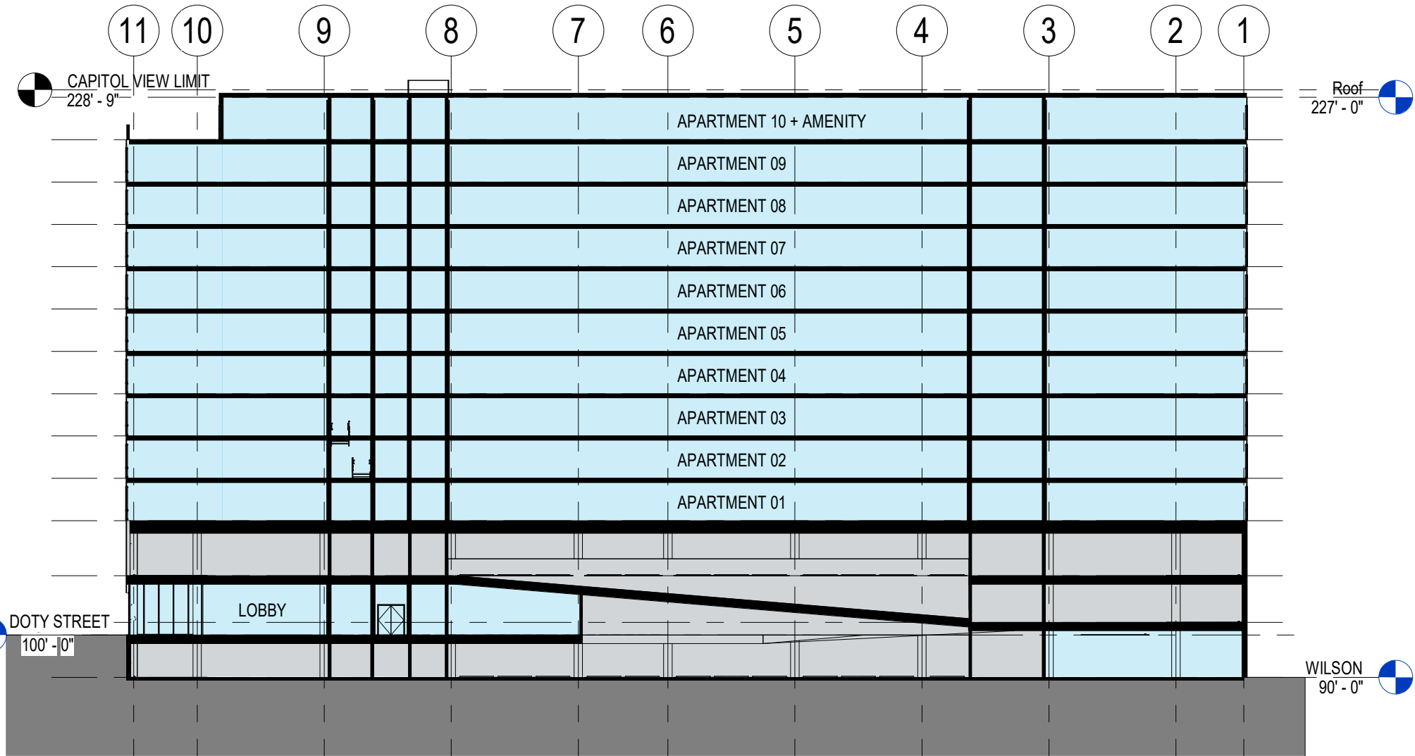
LONGITUDINAL SECTION
