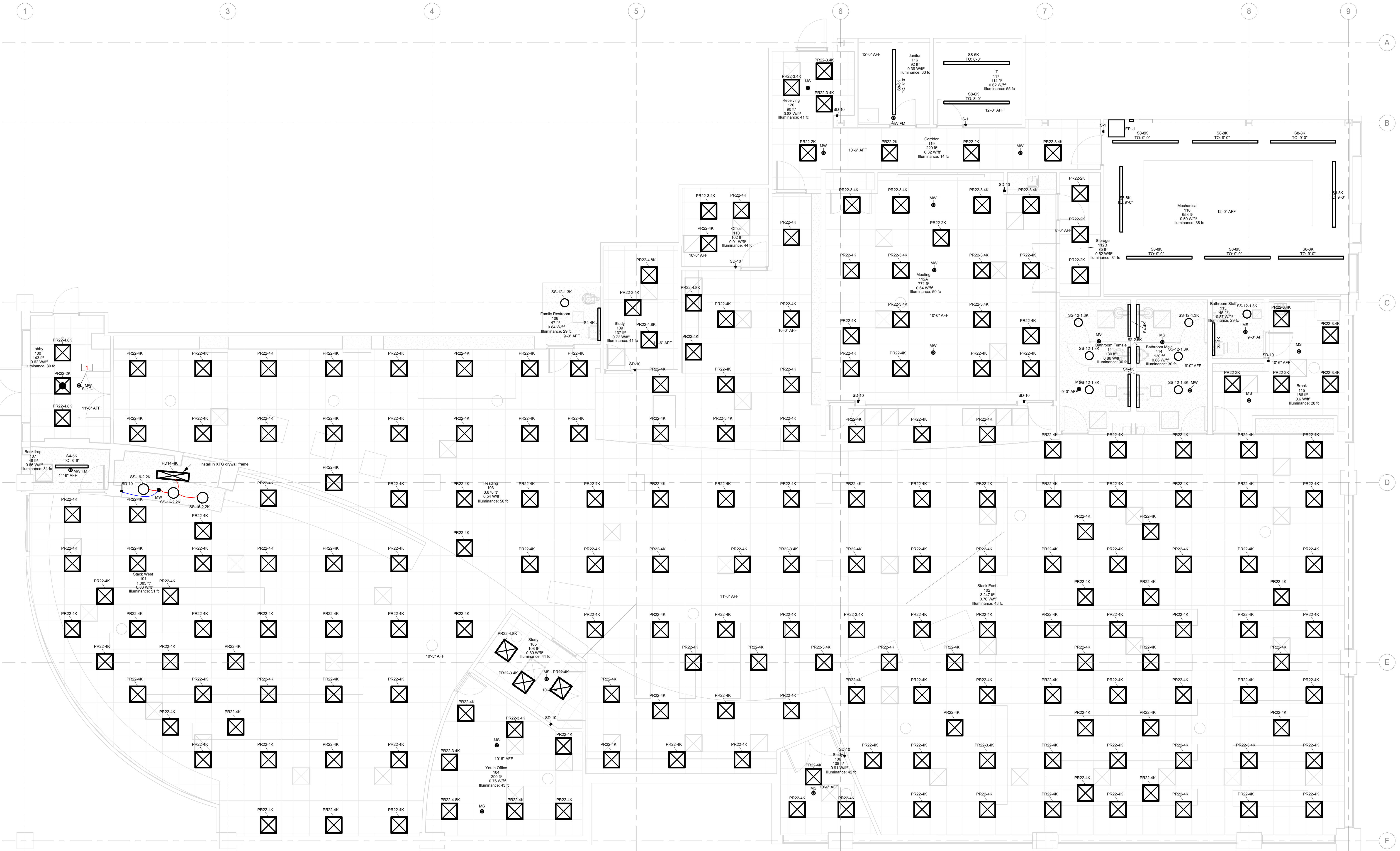
1 EL - Level 1 3/16" = 1'-0"
