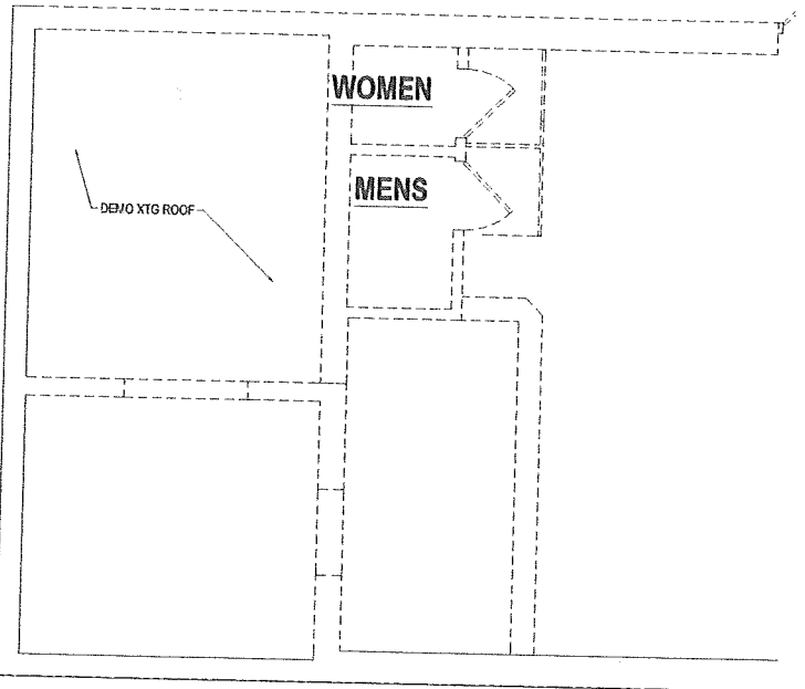
DEMO PLAN SCALE: 1/4" = 1'-0"
