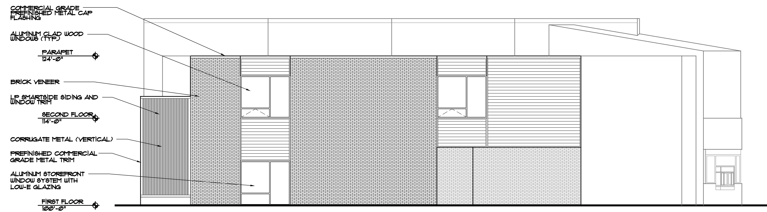
3 BACK ELEVATION A-2.1 SCALE: 1/8" = 1' - 0"
