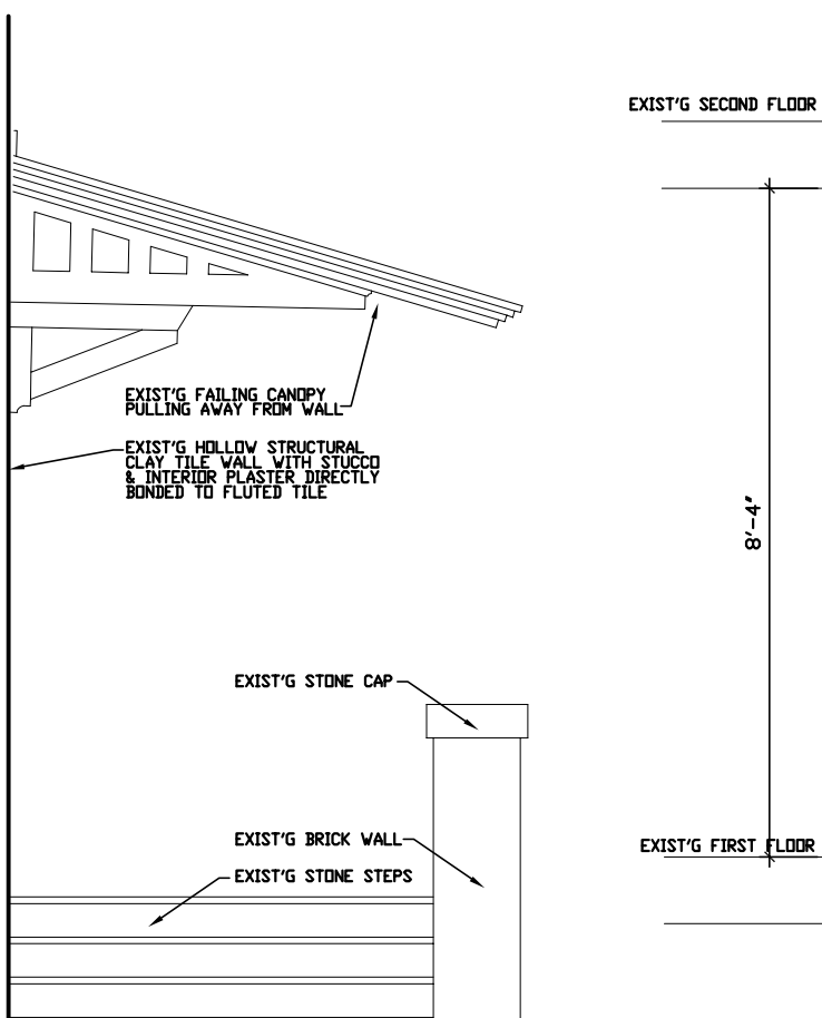
PORCH- SIDE ELEVATION SCALE: 3/8" = 1'-0" EXISTING
