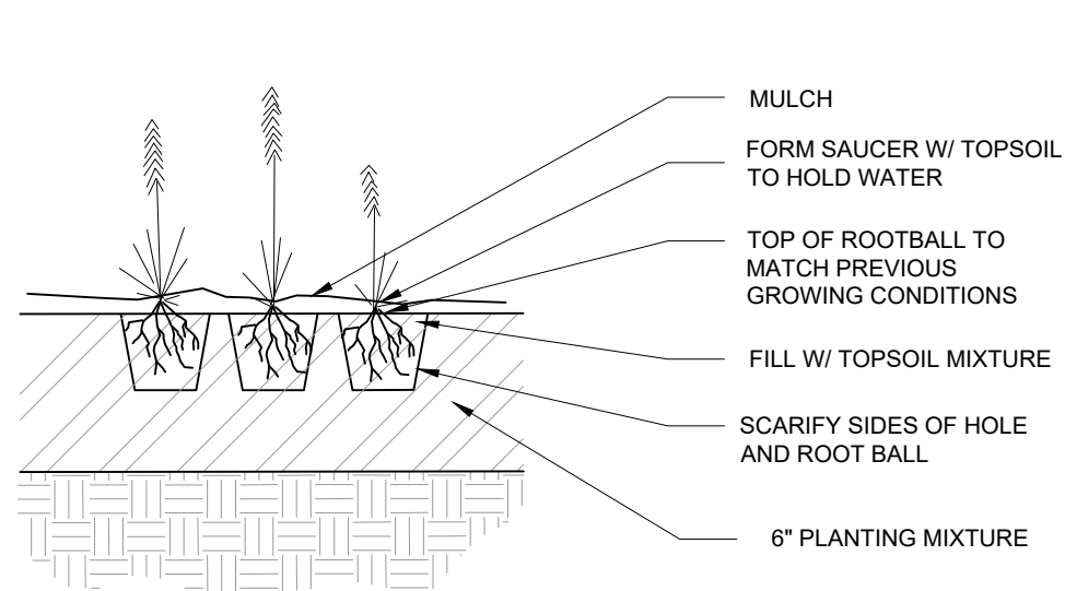
ORNAMENTAL GRASSES DETAIL (N.T.S.)
