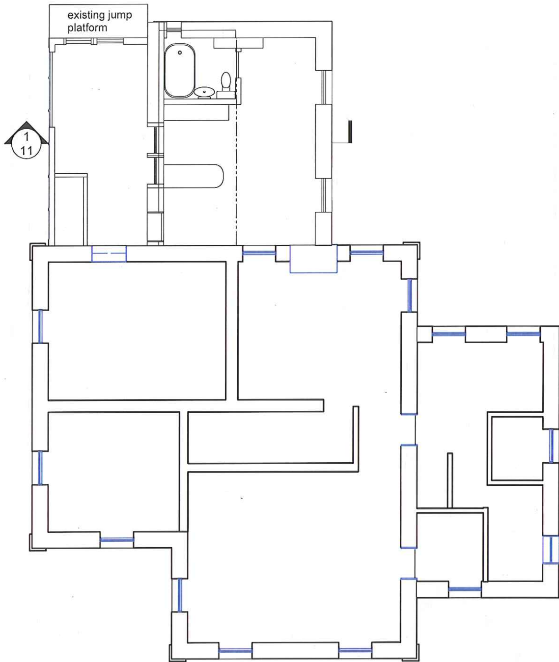
1 Floor Plan-2 3 Scale: 1/8" = 1'-0"
