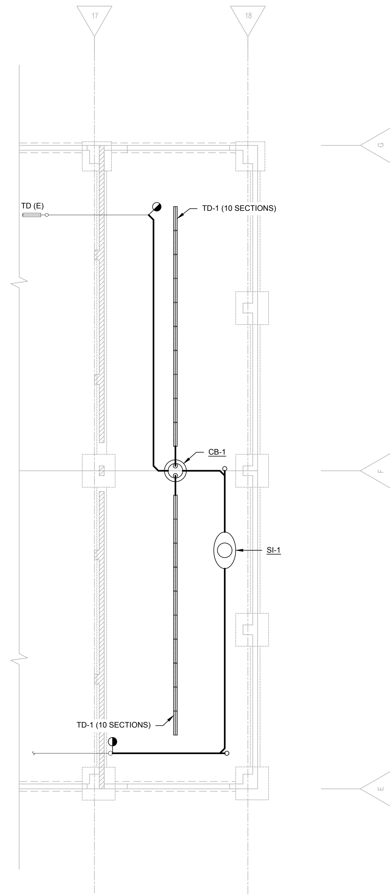
2 UNDERFLOOR PLAN - PLUMBING P200 SCALE: 1/8"=1'-0"
