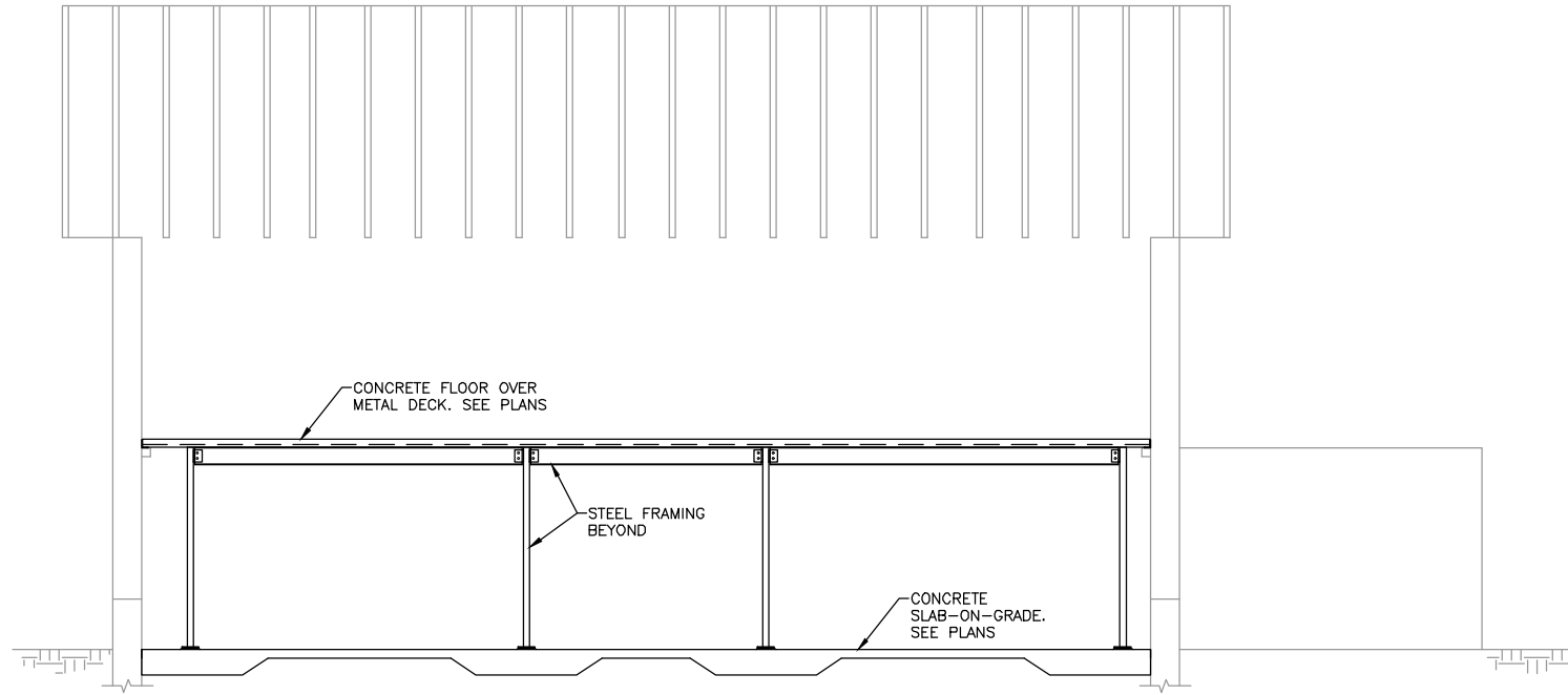
SECTION 2 AS3.1
