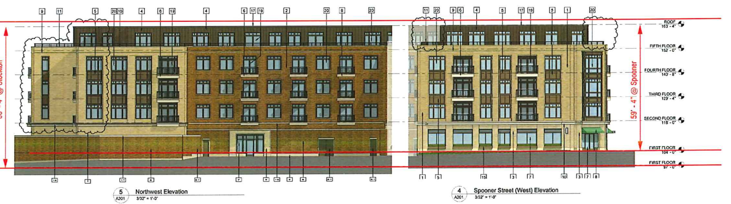
02.07.2018 Elevations
