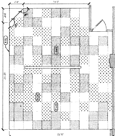
02 Carpet Pattern SCALE: 1/8" = 1'-0"
